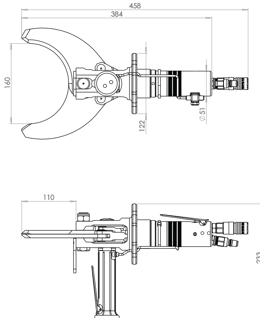
Maßskizze
