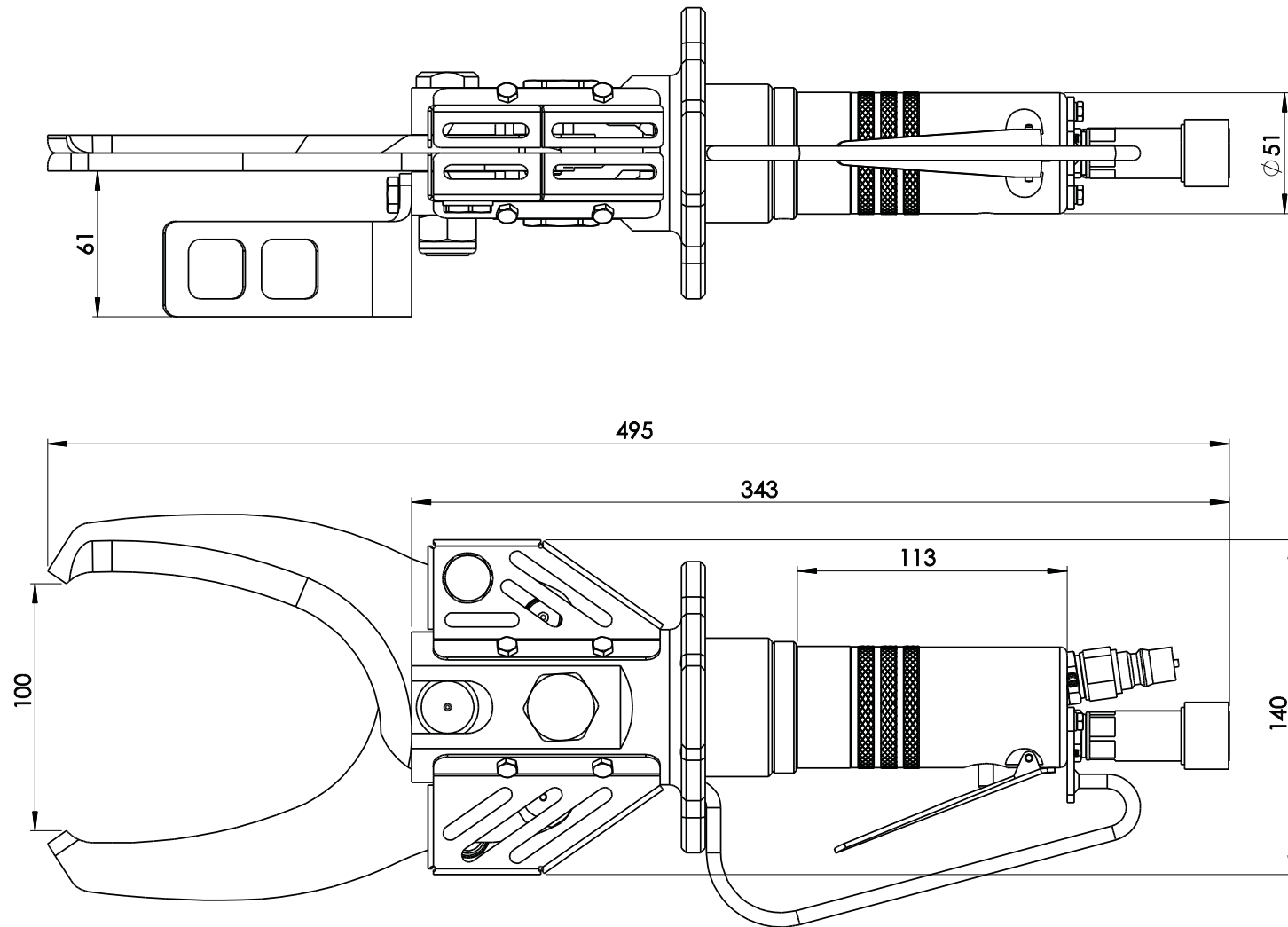
Maßskizze
