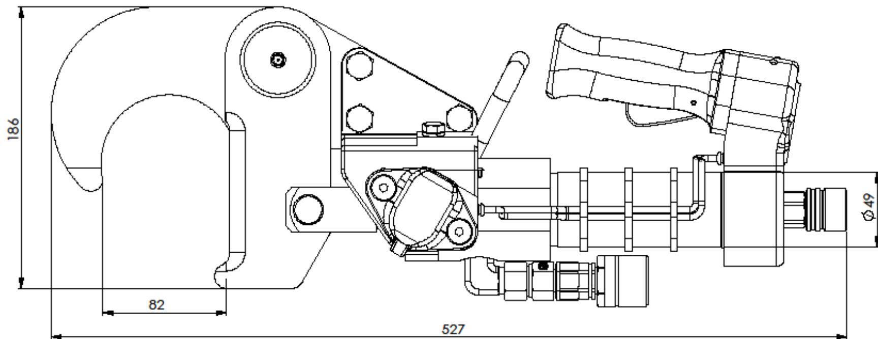
Maßskizze
