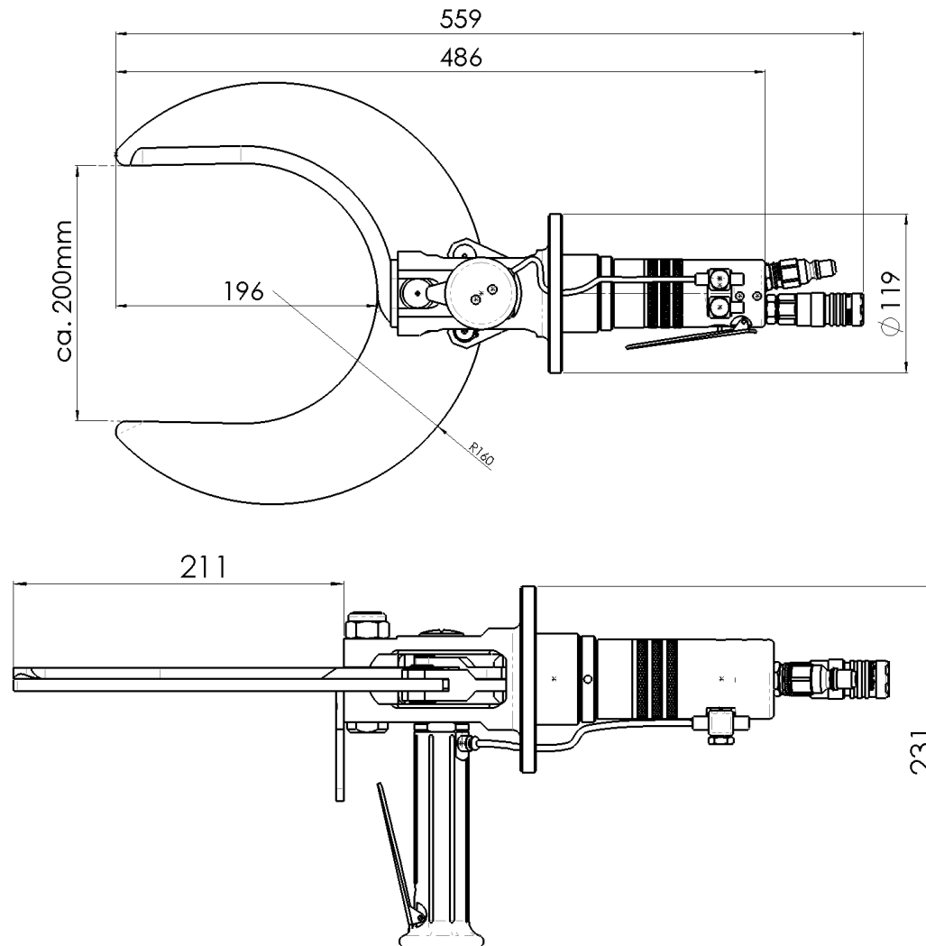
Maßskizze
