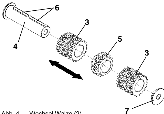
Abb. 4 Wechsel Walze (2)
