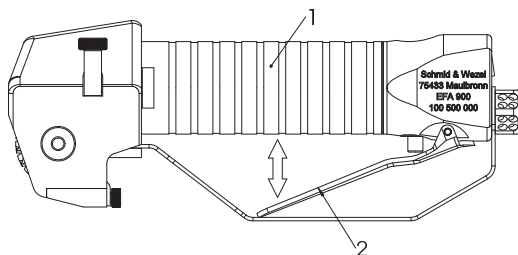
Abb. 2 Schalterbetätigung
