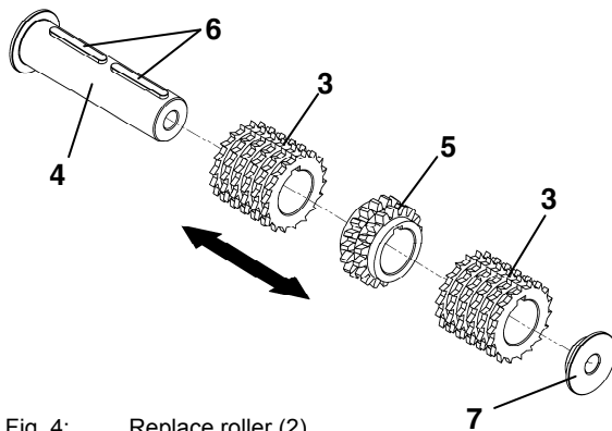
Fig. 4: Replace roller (2)
