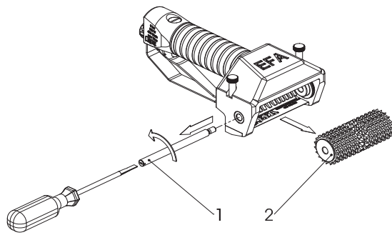
Fig. 3: Replace roller (1)
