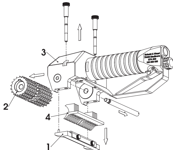
Abb. 8 Ausbau Reinigungskralle
