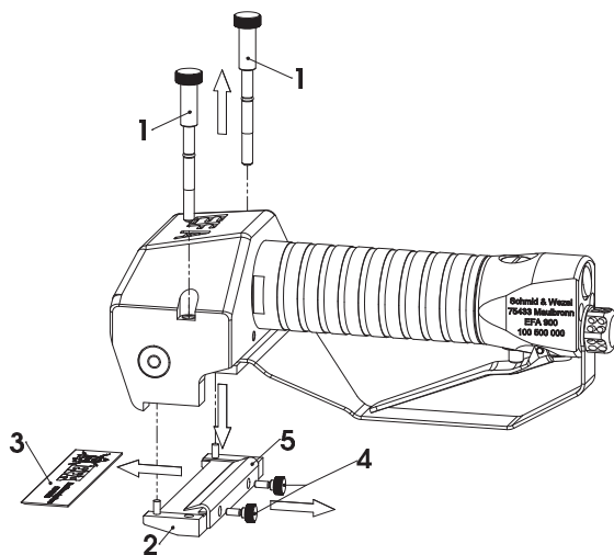
Abb. 6 Messerwechsel
