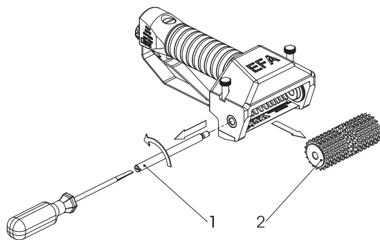
Abb. 3 Wechsel Walze (1)
