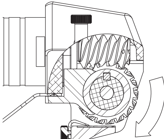
Abb. 5 Schnitt durch Walze, Zahnrichtung
